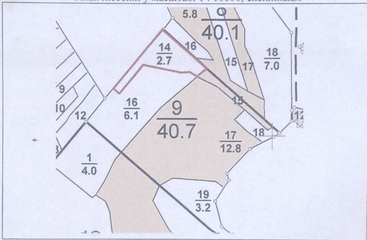
План лісосіки у масштабі 1 : 10000, експлікація
