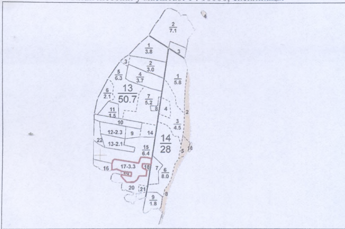
План лісосіки у масштабі 1 : 10000, експлікація
